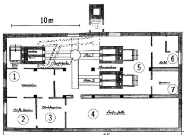
Plattegrond oorspronkelijke situatie Krematorium I Hoofdkamp. Van de lijkenkamer (4) werd later gezegd dat die als 'gaskamer' werd gebruikt. 1: Vestibule; 2. Autopsiekamer; 3. Wasruimte; 4. Lijkenopslag; 5. Ovenruimte; 6. Cokesopslag; 7. Urnenruimte.
