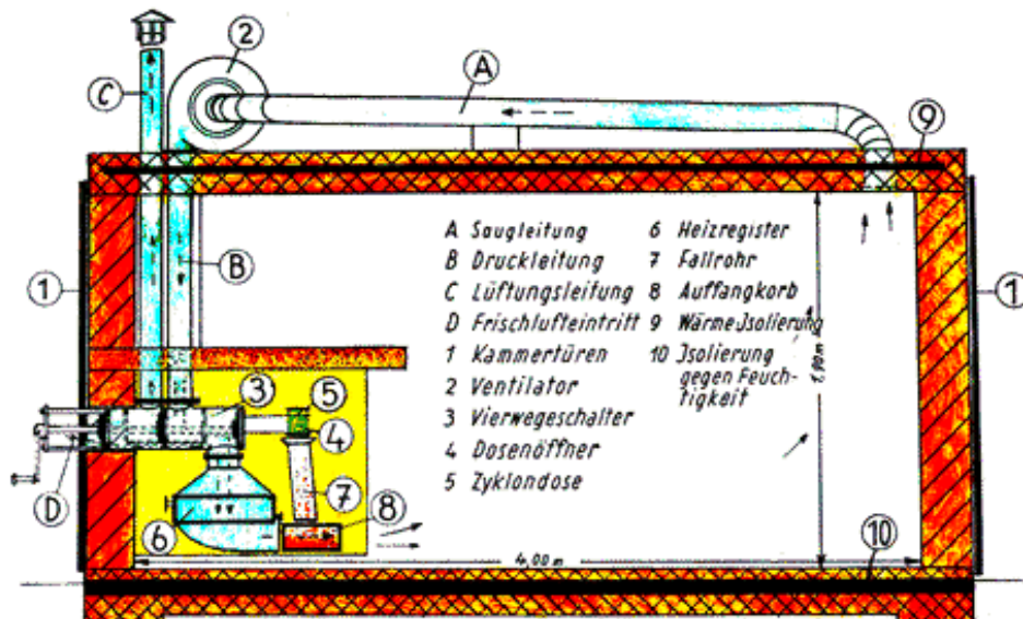
Doorsnedetekening installatie voor textielontluising in Duitse concentratiekampen. Zoals te zien, is de luchtcirculatie tegengesteld aan die van de 'gaskamers': aanvoer bij de vloer en afzuiging bij het plafond!
