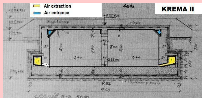
Schema zijaanzicht Krema's II en III: luchttoevoer plafond (blauw), afzuiging vloer (geel). Normaal voor lijkenkamers, averechts voor gaskamers. 1414
