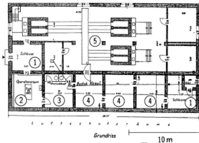
Plattegrond na tussentijdse buitengebruikstelling en verbouwing tot schuilkelder met operatieruimte, tussenmuren en verspringende deuren voor betere luchtdrukweerstand.
