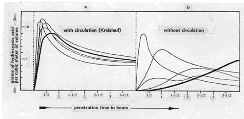
Verdamping/verspreiding Zyklon-B met en zonder circulatie.
